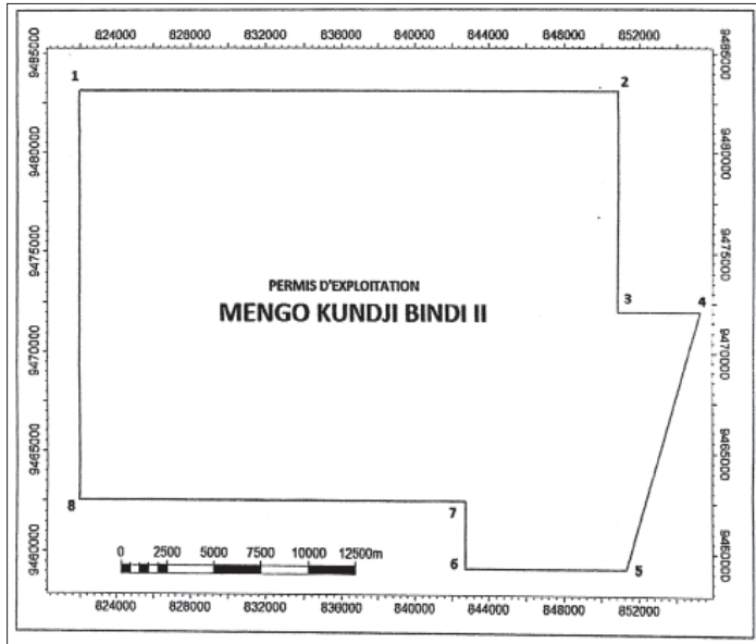
Figure 89 : Plan de position du permis d'exploitation "Mengo Kundji Bindi II"
